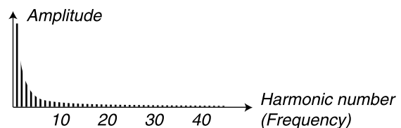
Lo spettro della frequenza del segnale a dente di sega
