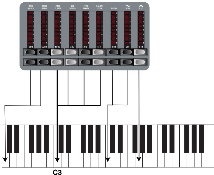
Nella figura sopra è stato scelto C3 come nota di riferimento. I quattro selettori ‘Register’ corrispondono all’armonico fondamentale (ma con differenti caratteristiche tonali). Le frecce puntano alle rispettive note che ogni Drawbar rappresenta quando C3 viene suonato.
